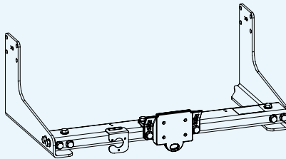
Systeem voor bestelwagen met grote opstap
